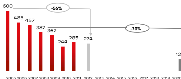
Emissões específicas de CO 2 do Grupo EDP (gCO 2 /kWh) e objectivos de redução
